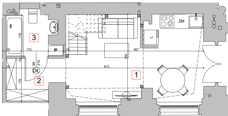
POZIOM PARTERU
