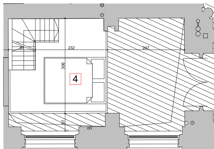
POZIOM ANTRESOLI
