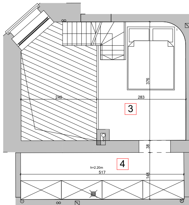
POZIOM ANTRESOLI
