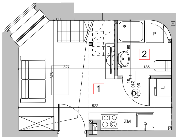
POZIOM PARTERU
