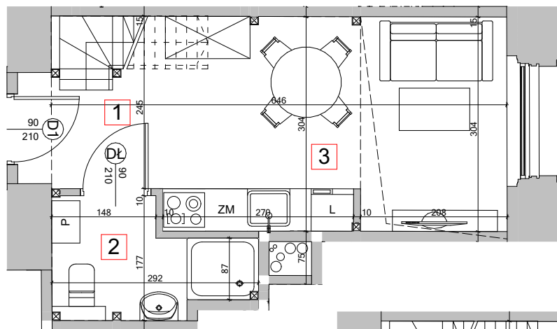
POZIOM PARTERU
