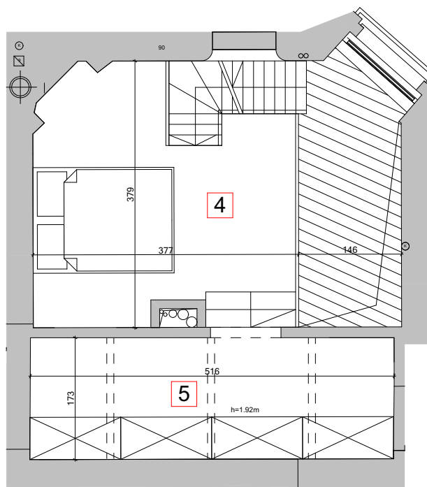
POZIOM ANTRESOLI
