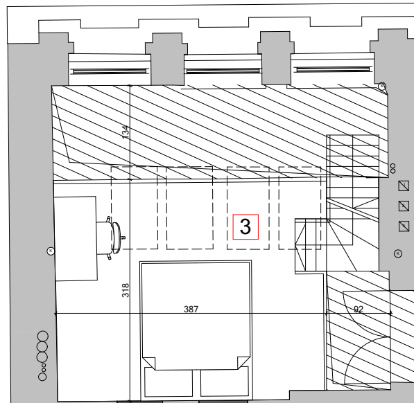
POZIOM ANTRESOLI
