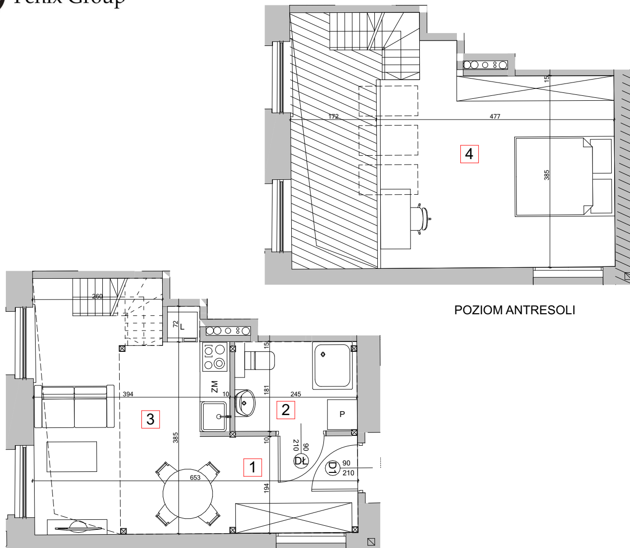
POZIOM PIĘTRA I
