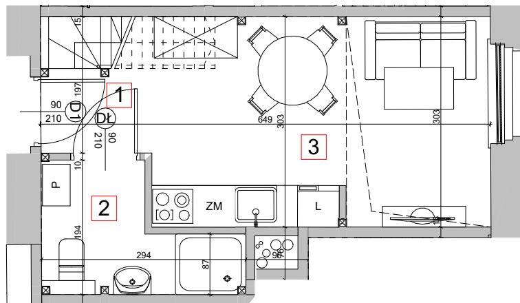
POZIOM PIĘTRA I
