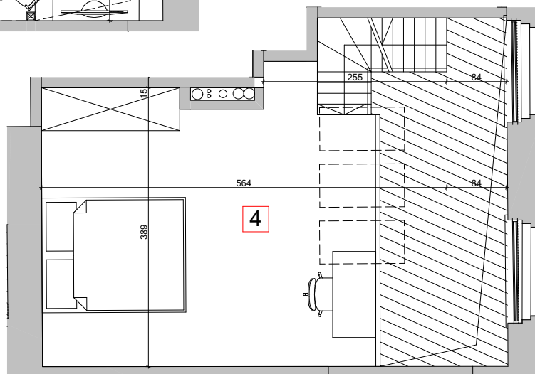
POZIOM ANTRESOLI
