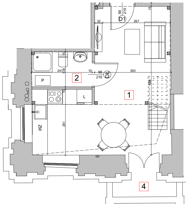
POZIOM PIĘTRA I
