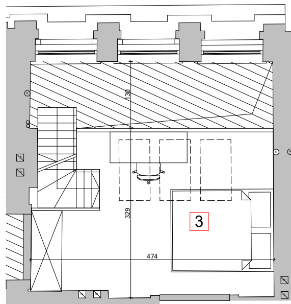
POZIOM ANTRESOLI
